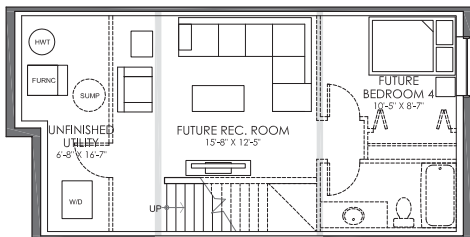
OPTIONAL BASEMENT PLAN
